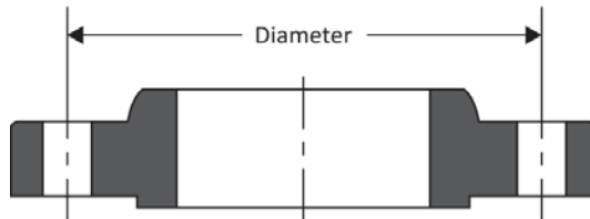
Bolt Circle
